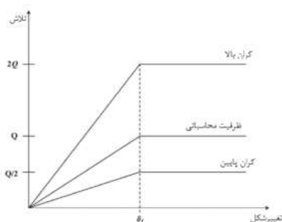
شکل پ ۴-۴ رفتار دوطرفی معادل با رفتار غیرخطی فنرهای پی
