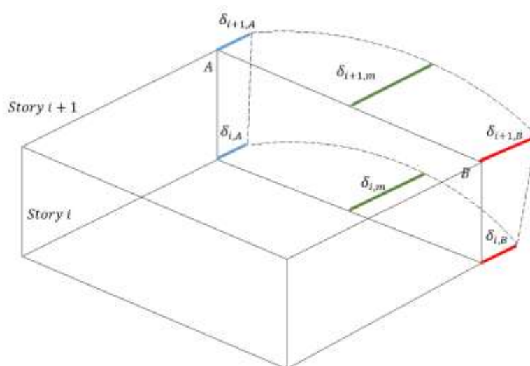
شکل پ ۲-۳ پارامترهای جابجایی مورد نیاز برای بررسی صلبیت دیافراگم
