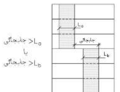
پ - نامنظمی قطع داخل صفحه
