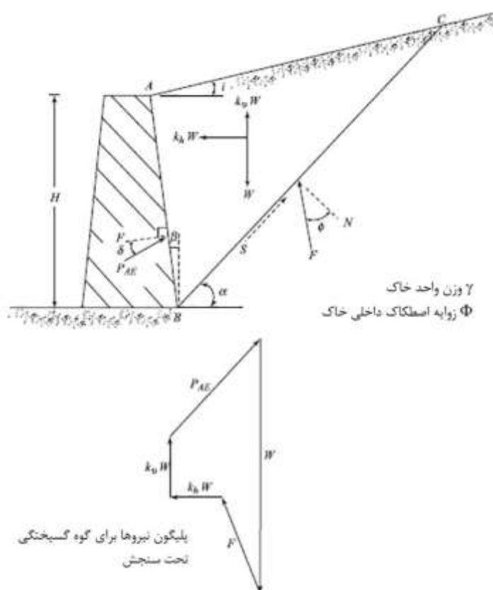
شکل پ ۶-۹ نحوه محاسبه نیروی محرک زلزله (معادله مونونوبه-اکابه)
