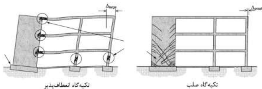
(ب) تکیه‌گاه انعطاف پذیر
