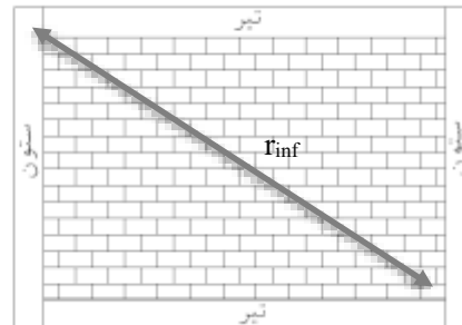
(الف) دیوار با عملکرد میانقابی
